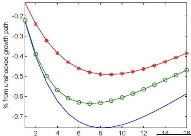
A: output
